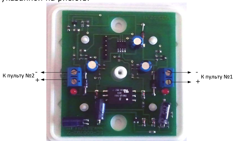
Рисунок 6.1. Внешний вид GC-0002D1 (со снятой крышкой)
